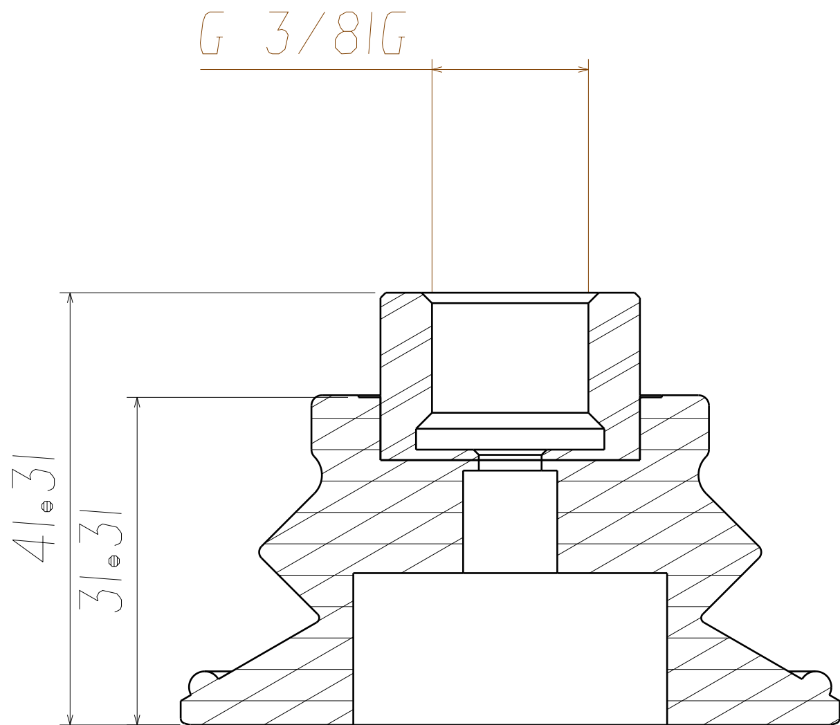
剖视图A-A 缩放: 2:1
