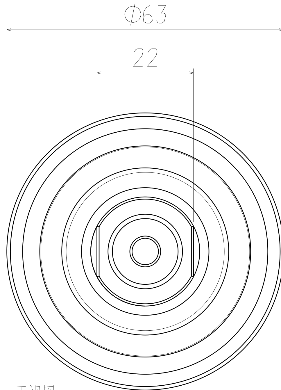
正视图 缩放: 2:1
