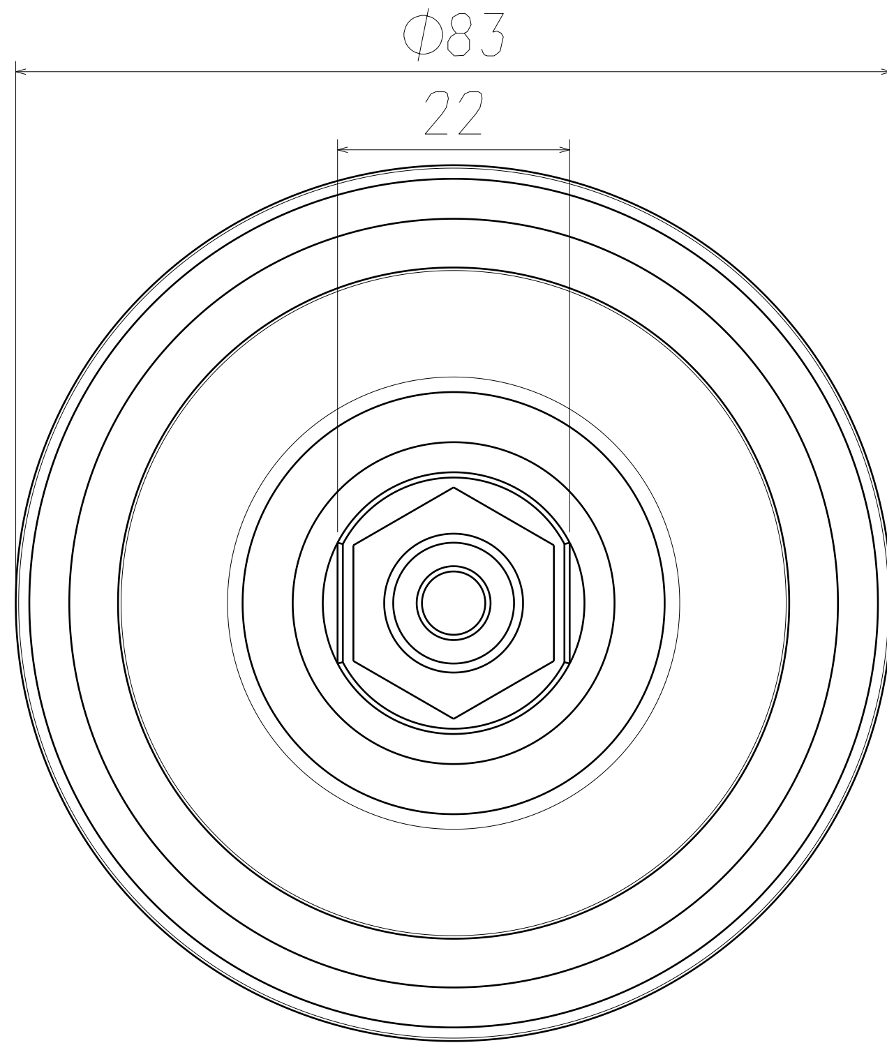
正视图 缩放: 2:
