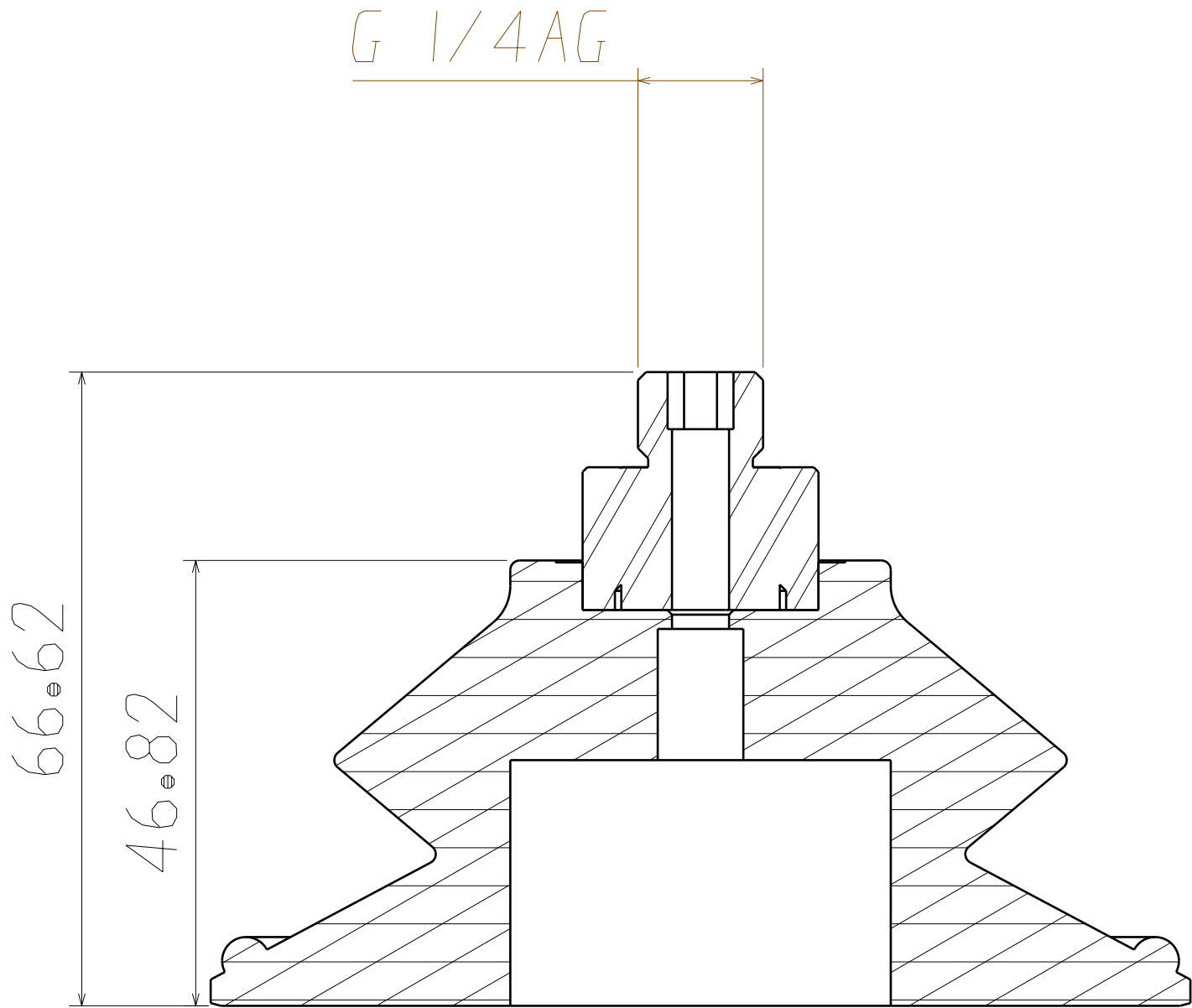
剖视图A-A 缩放：3:2
