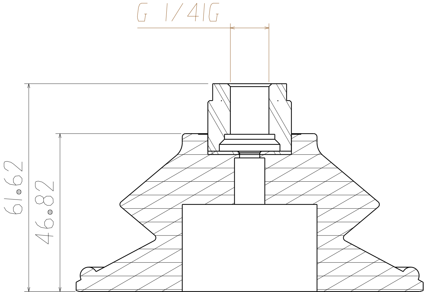
剖视图A-A 缩放: 3:2
