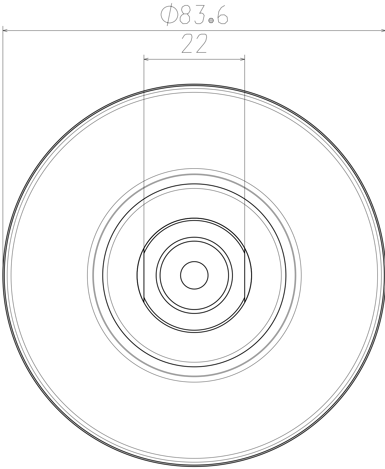
正视图 缩放：2:1
