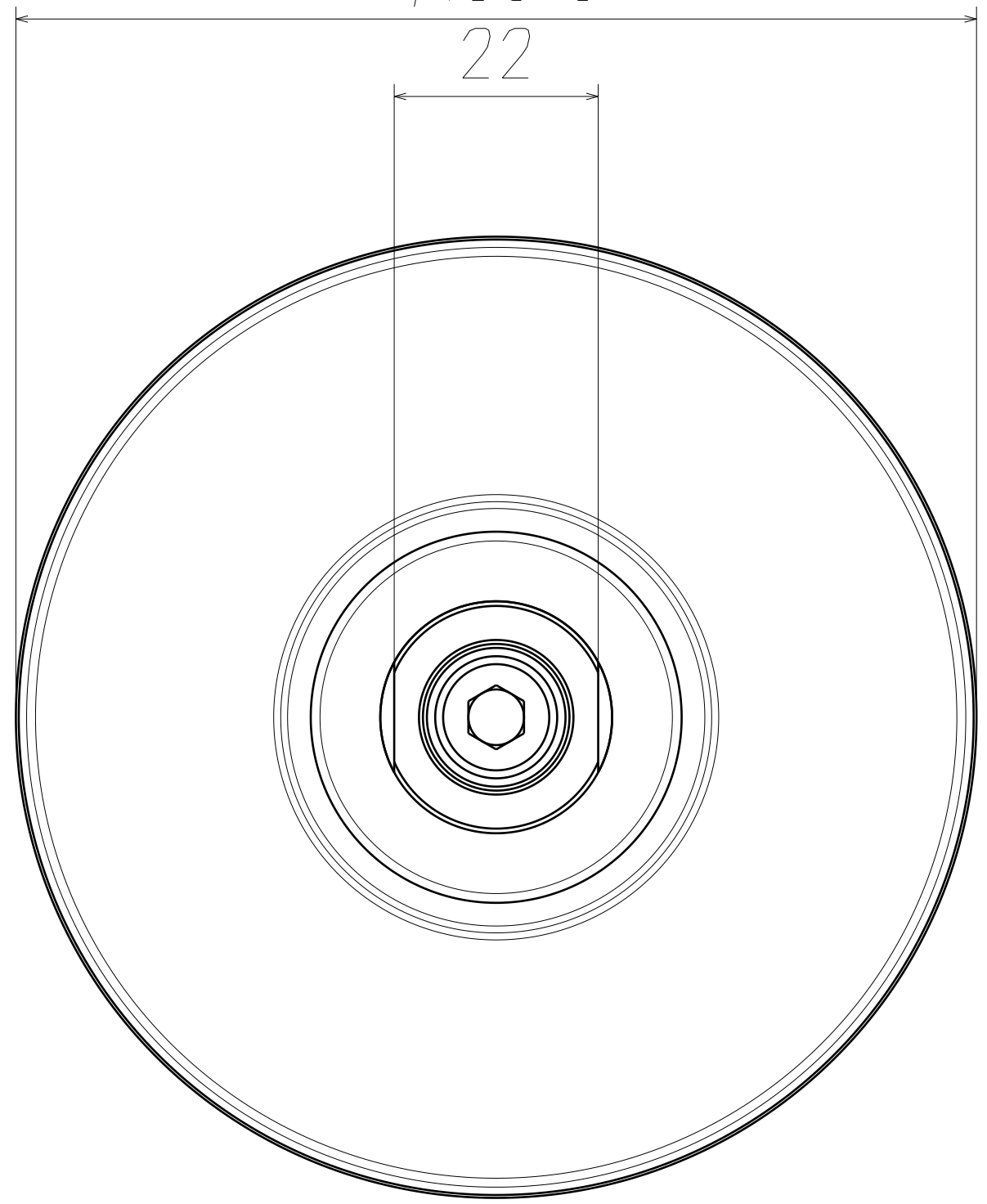
正视图 缩放: 3:2
