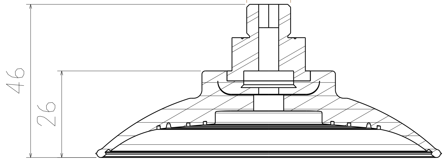
剖视图A-A 缩放: 3:2
