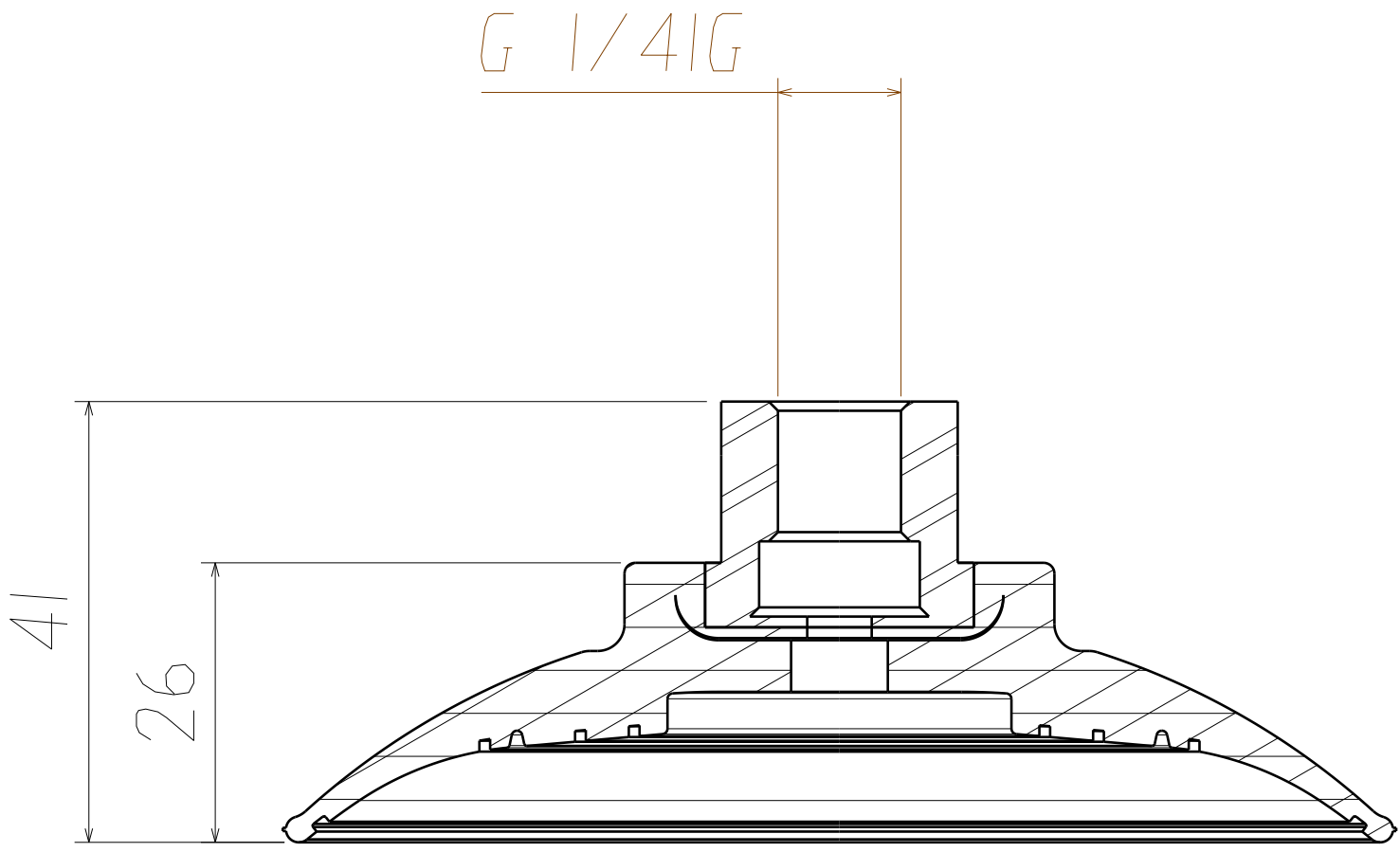
剖视图A-A 缩放: 3:2
