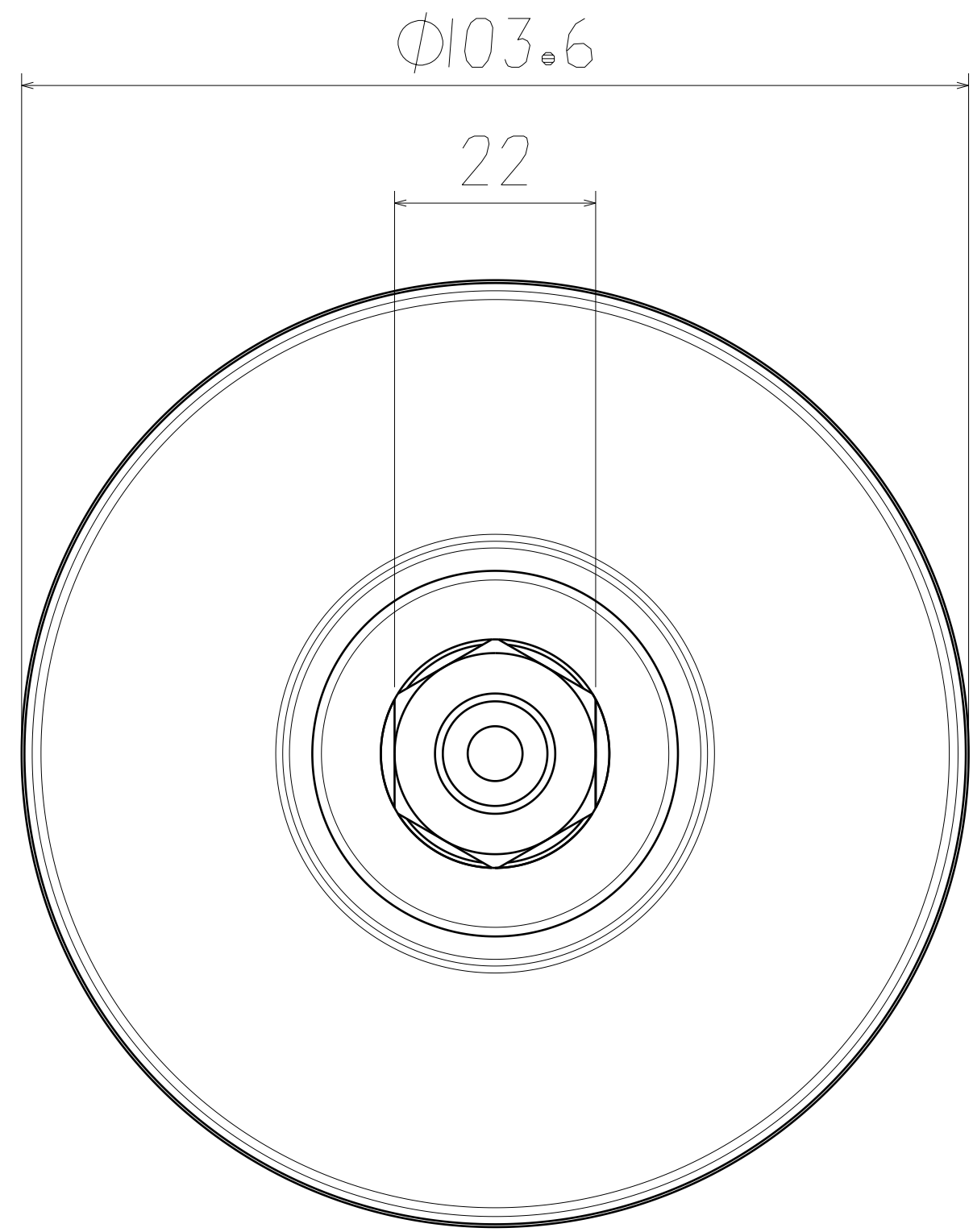
正视图 缩放: 3:2
