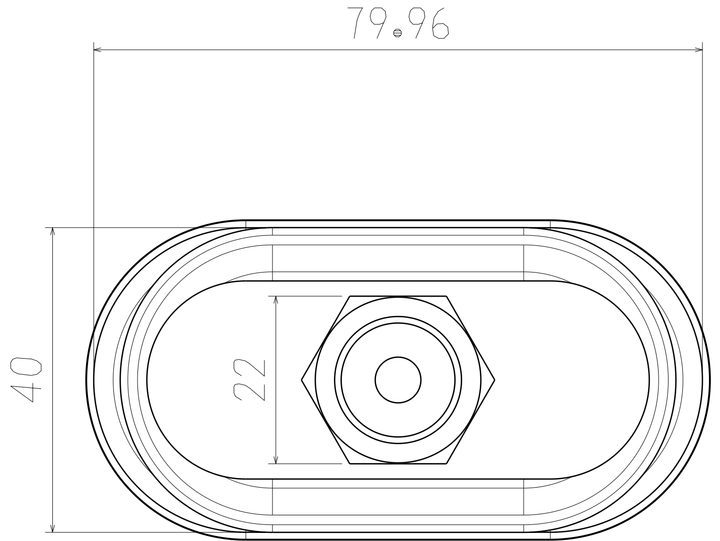
正视图 缩放: 2
