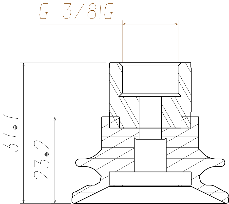
剖视图A-A 缩放: 2
