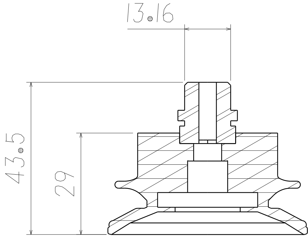
剖视图A-A 缩放: 3:2
