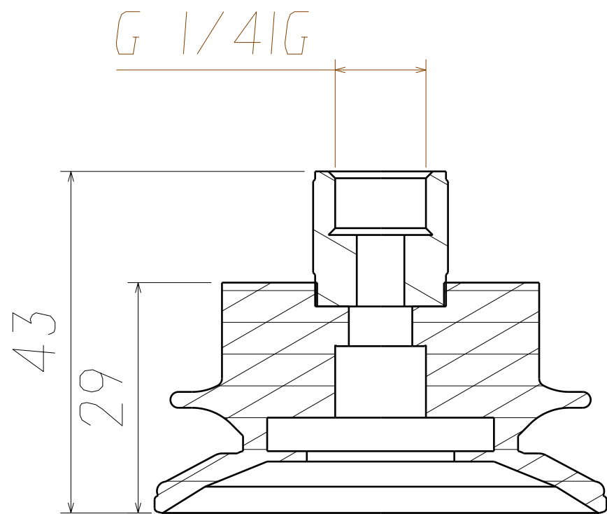
剖视图A-A 缩放：3:2
