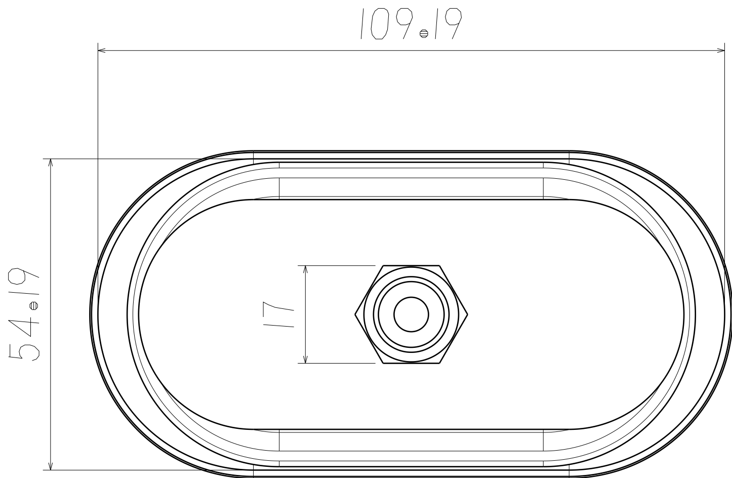
正视图 缩放：3:2
