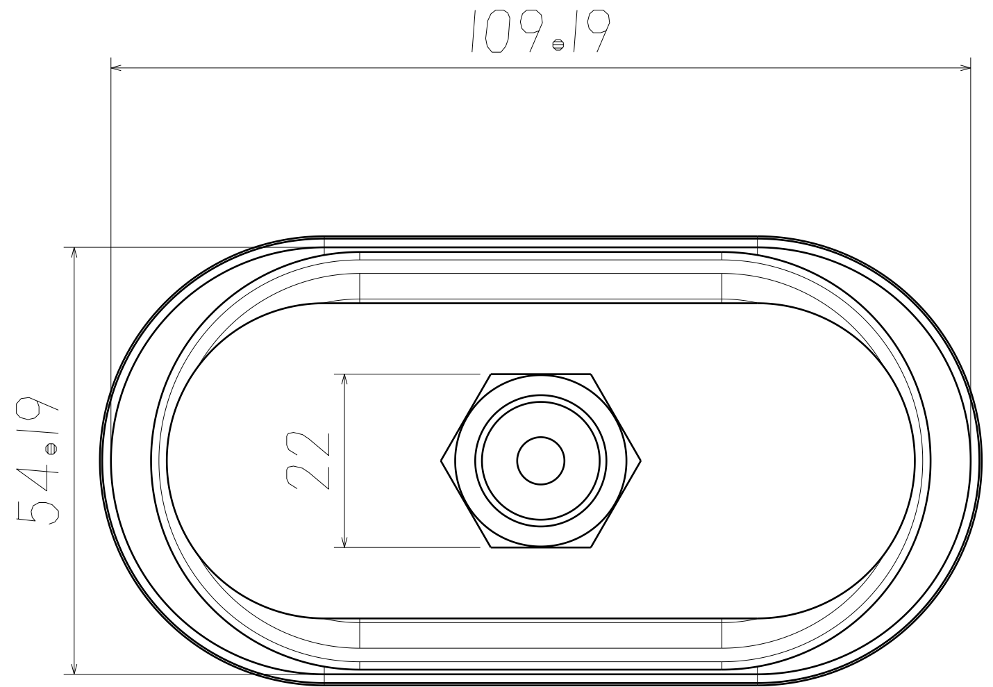
正视图 缩放: 3:2
