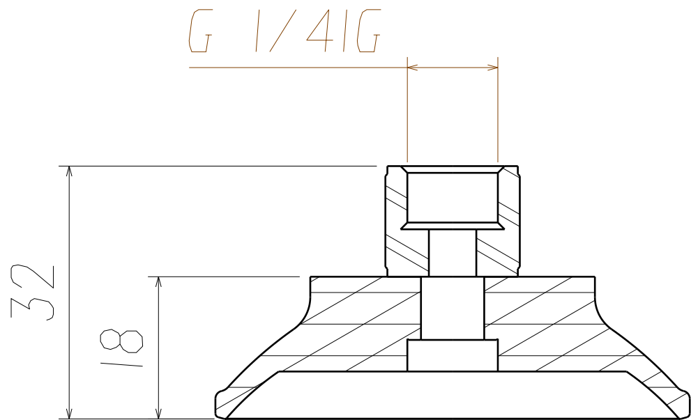
剖视图A-A 缩放: 3:2
