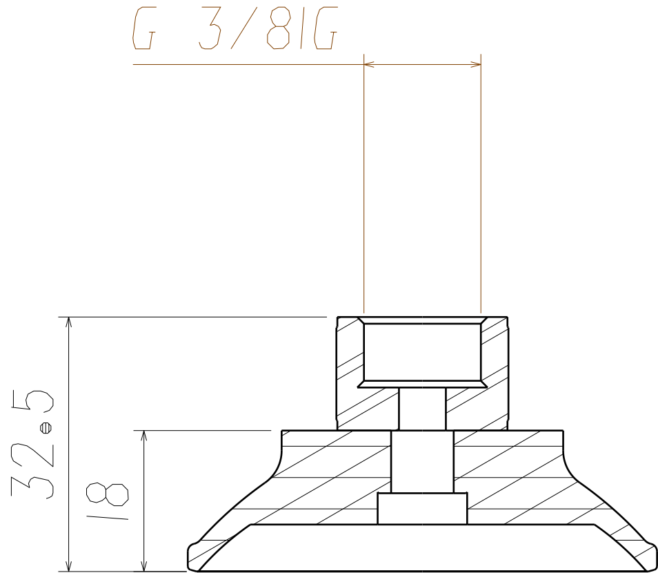
剖视图A-A 缩放: 3:2
