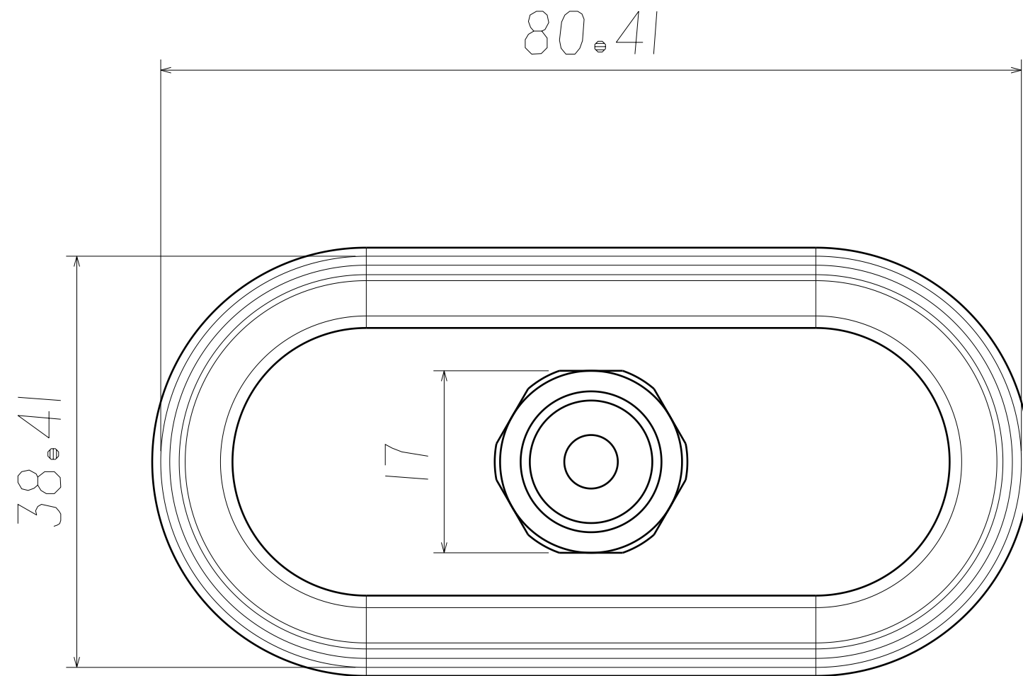
正视图 缩放: 2:1
