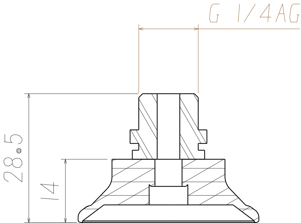
剖视图A-A 缩放: 2:1
